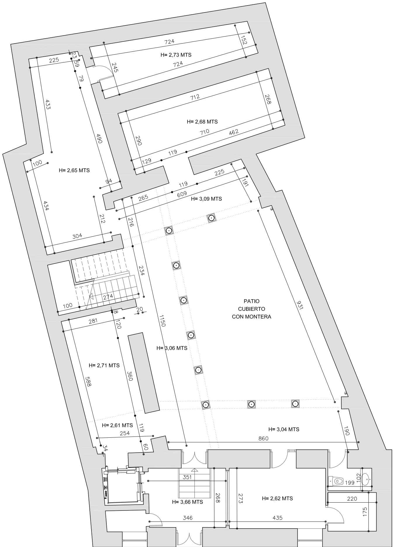
PLANTA BAJA
